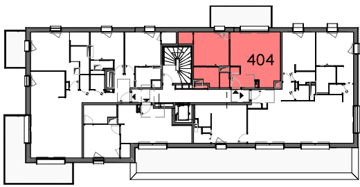
Plan de repérage appartement A-404
